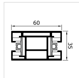
Odsazená vodící lišta na sloupek FS ZT60VT
