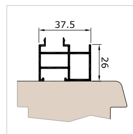
Adaptérová lišta ADS26Z
