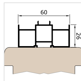
Adaptérová lišta ADS26ZK
