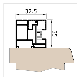
Vodící lišta FS Z37VP, zaomítací varianta
