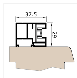
Vodící lišta FS Z37V
