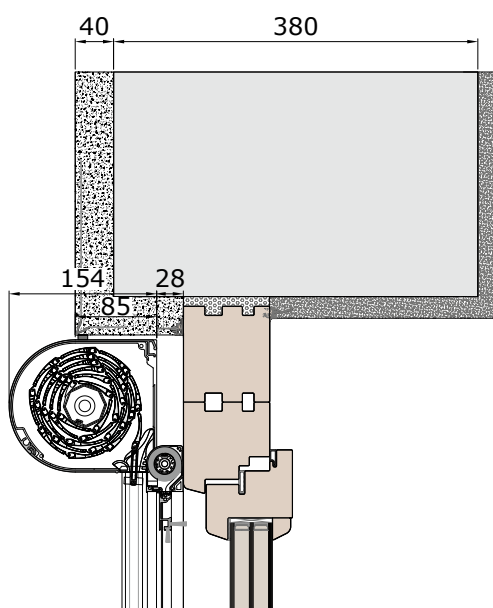
S rámovým zdvojením. VORO BRAVO s kombinovanou rolo sítí.
