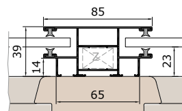
Sloupek s vodicí lištou KF85V
