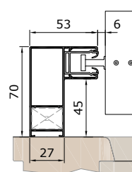
Vodicí lišta ED53V
