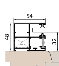
Vodicí lišta KR54V
