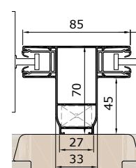
Sloupek s ED85V
