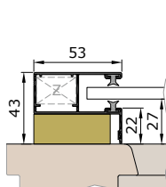
Termicky oddělená vodicí lišta K53VT
