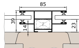
Sloupek s vodicí lištou KE85V
