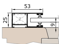
Vodicí lišta K53V
