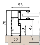
Vodicí lišta KD53SA
