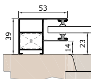
Vodicí lišta KE53V pro renovace
