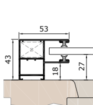
Vodicí lišta KA53V
